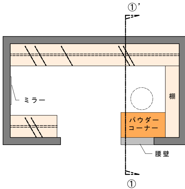
平面プラン
